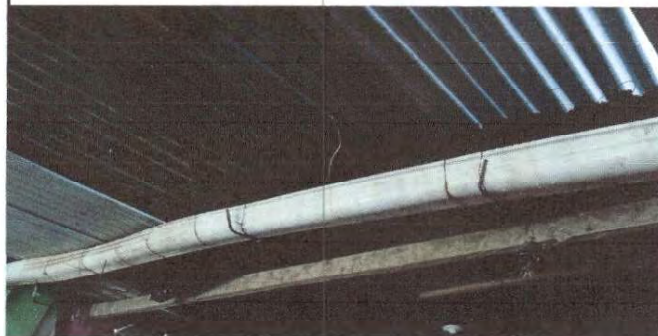
Foto 10: Sustitución de canales y bajada de agua aula 2.
